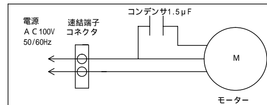
結線図
