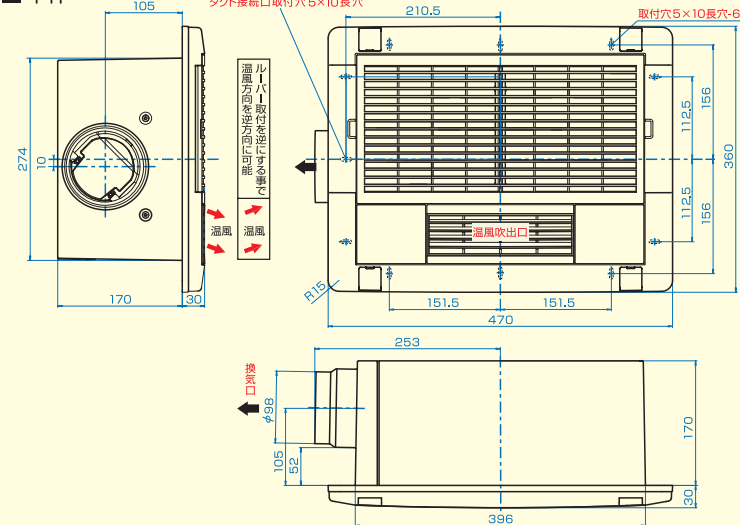
UB-231SHA (単位:mm)
