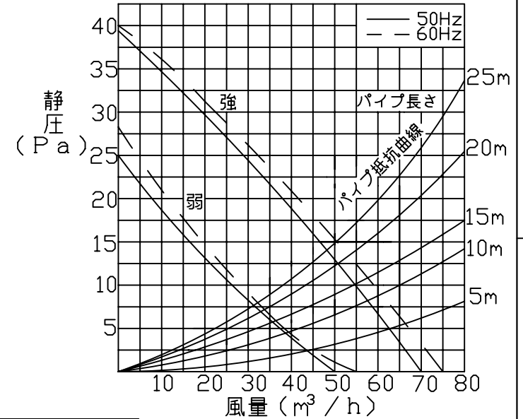
静圧曲線 抵抗曲線はVP管φ100の場合
