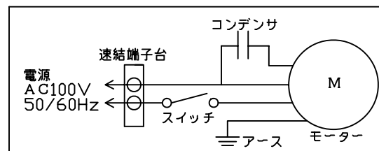
■結線図
