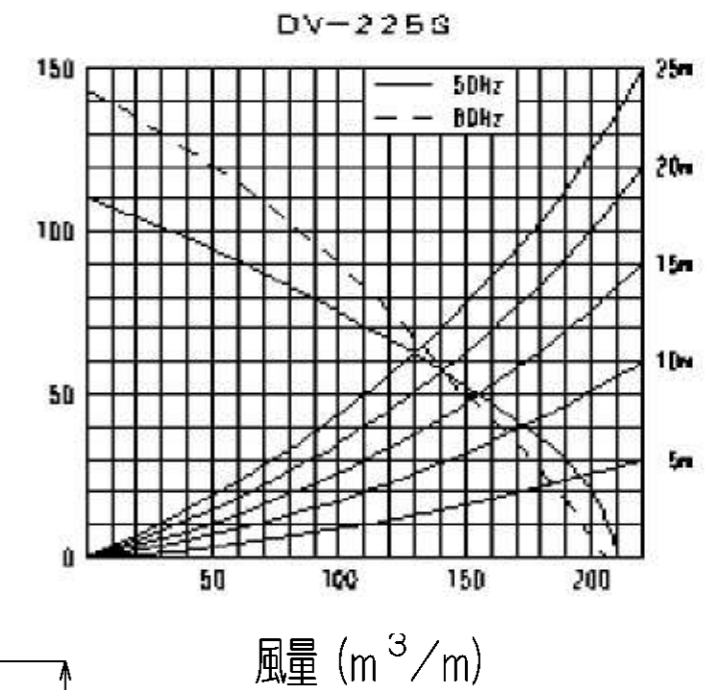
Pa DV-225S静圧曲線表
