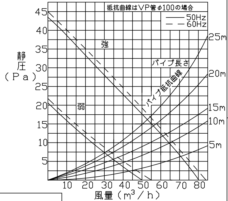
静圧曲線
