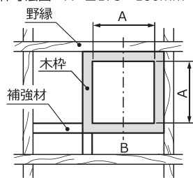
取付枠寸法図 A=□175~180mm
