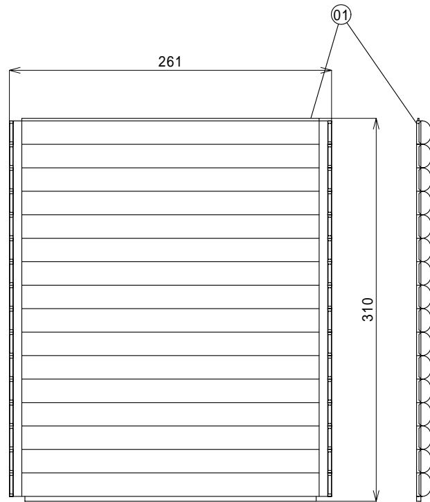
パネル
